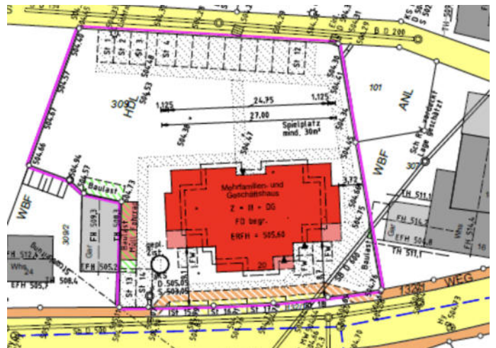
Lageplan des Bauvorhabens
